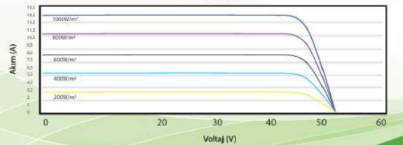
I-V Eğrileri (560W)
